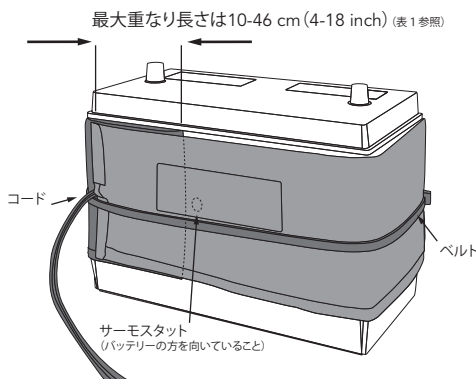
図1 バッテリーカバーの取り付け (最大重なり推奨値)
